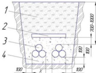
Рисунок 1. Прокладка кабелей 6 - 35 кВ в траншее, расстояние между кабельными линиями при параллельной прокладке в земле. 1 - засыпной грунт; 2 - железобетонная плита; 3 - кабели 6 - 35 кВ; 4 - песчано-гравийная смесь или мелкий грунт. (Для кабелей 6 - 10 кВ расстояние X > 100 мм; для 20 - 35 кВ X > 250 мм)
