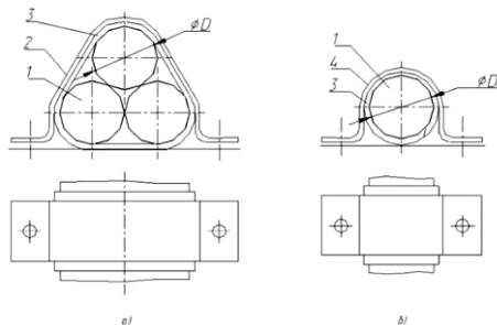
Рисунок 2. Варианты крепления кабеля на металлоконструкциях. 1 - кабели, 2 - металлический хомут (скоба), 3 - прокладка из эластичного материала, 4 - металлический хомут (скоба) из немагнитного материала
