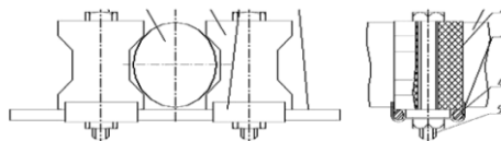
Рисунок 4. Вариант крепления кабеля с помощью клиц. 1 - кабель, 2 - клица, 3 - оцинкованная скоба, 4 - несущая арматура, 5 - болтовое соединение
