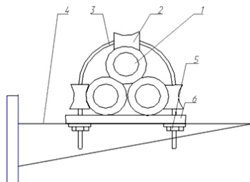
Рисунок 3. Вариант крепления кабеля с помощью клиц (треугольник). 1 - кабель, 2 - клица, 3 - оцинкованная скоба, 4 - кабельная палка, 5 - гайка, 6 - пластина
